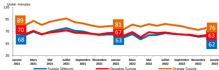
Evolution du trafic voix mobile off-net mensuel moyen par abonnement par opérateur
